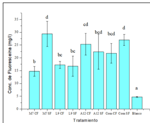
Figura 1.- Medida de la actividad enzimática FDA. Letras diferentes indican diferencias significativas entre los tratamientos ( p < 0,05 ).
