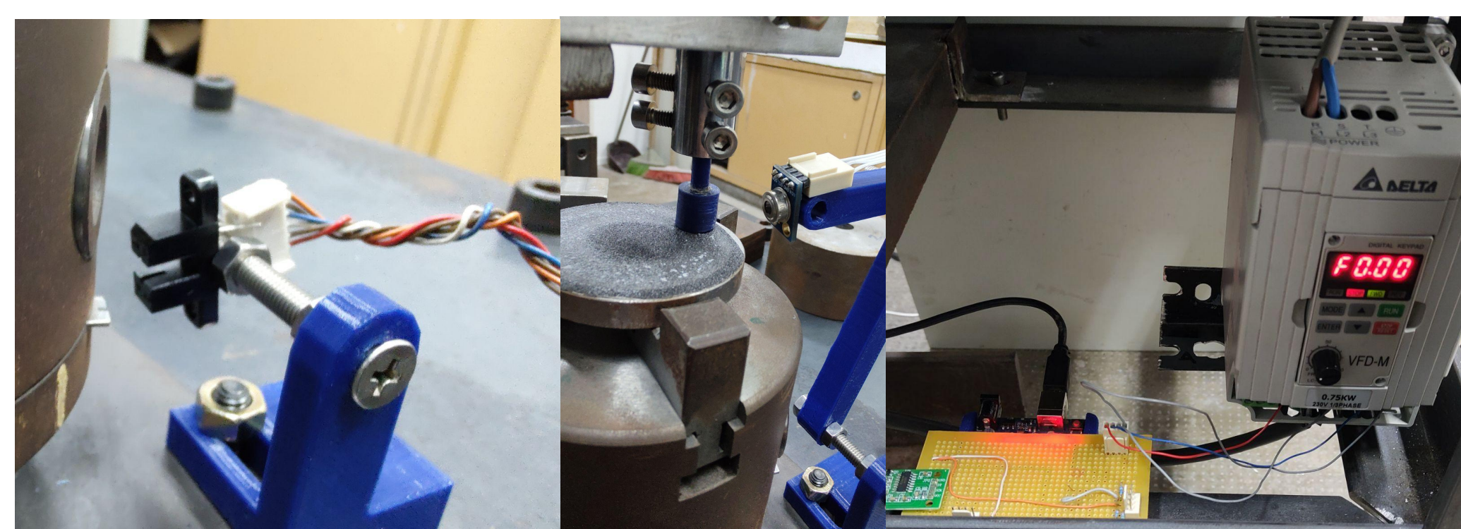
(a) Sensor de vueltas (b) Sensor de temp. (c) UC y Variador de F Figura 3. Tribómetro Pin-on-Disk del LEDFS
