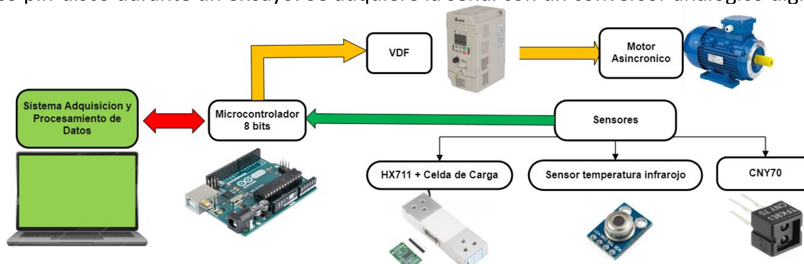
Figura 2. Diagrama general del sistema de adquisición y control
