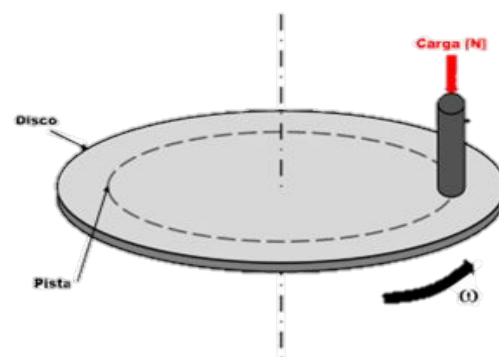
Figura 1. Esquema de funcionamiento ensayo Pin-on-Disk
