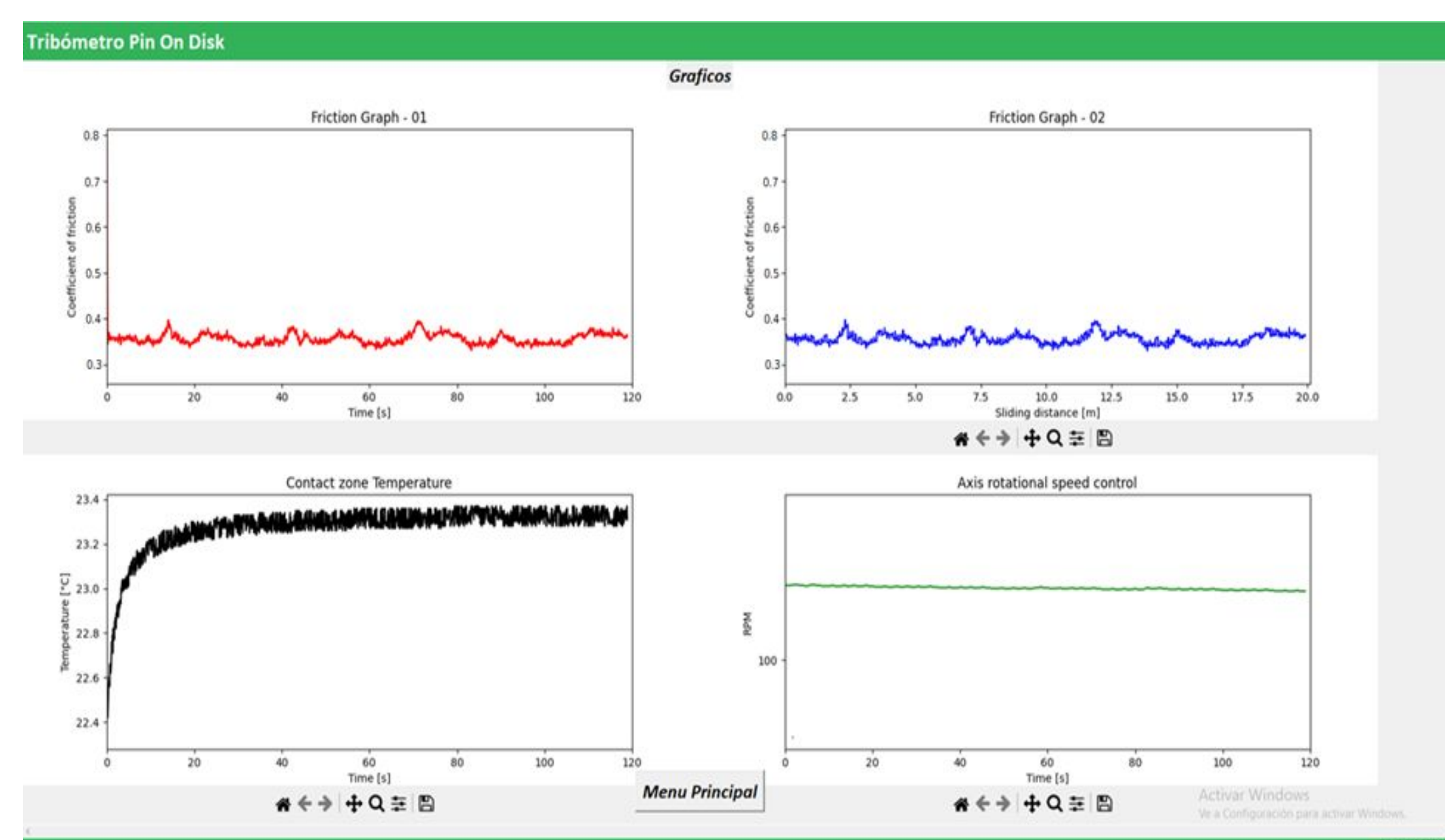
Figura 4. Captura de pantalla de un ensayo controlado y adquirido por el software
