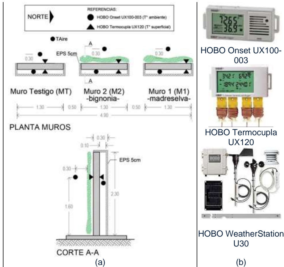
Figura 4. Casos de estudio: localización de sensores (a) y equipamiento (b).
