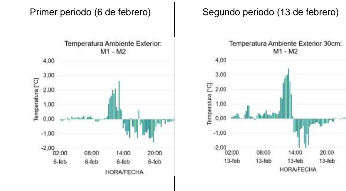
Figura 10. Diferencial hora a hora de la temperatura ambiente exterior a 0,30 m.
