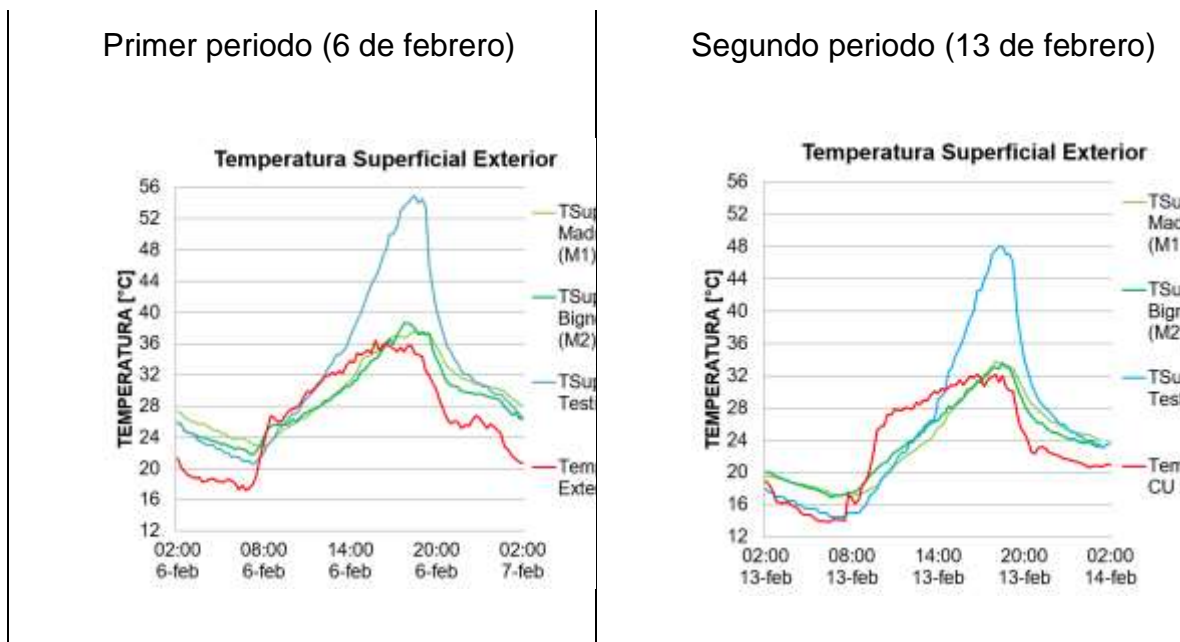
Figura 11. Temperatura superficial exterior.
