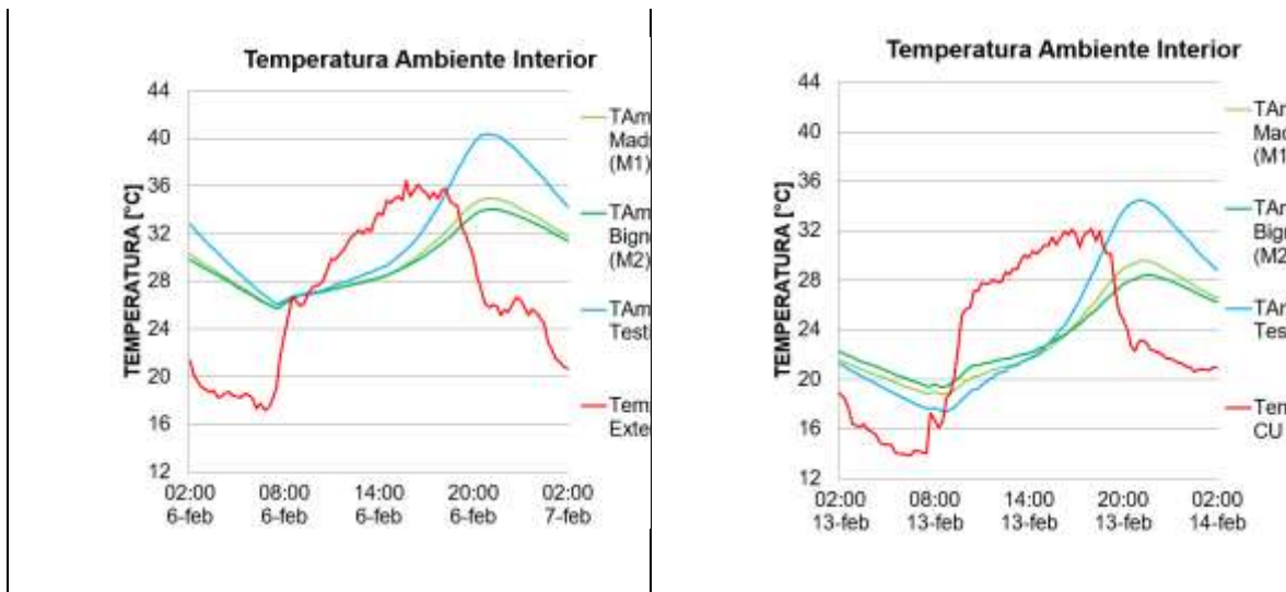
Figura 15. Temperatura ambiente interior.
