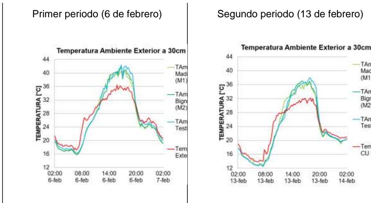
Figura 9. Temperatura ambiente exterior a 0,30 m.
