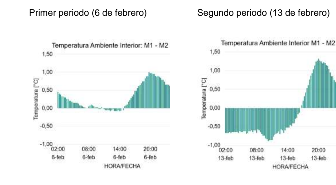
Figura 16. Diferencial hora a hora de la temperatura ambiente interior.
