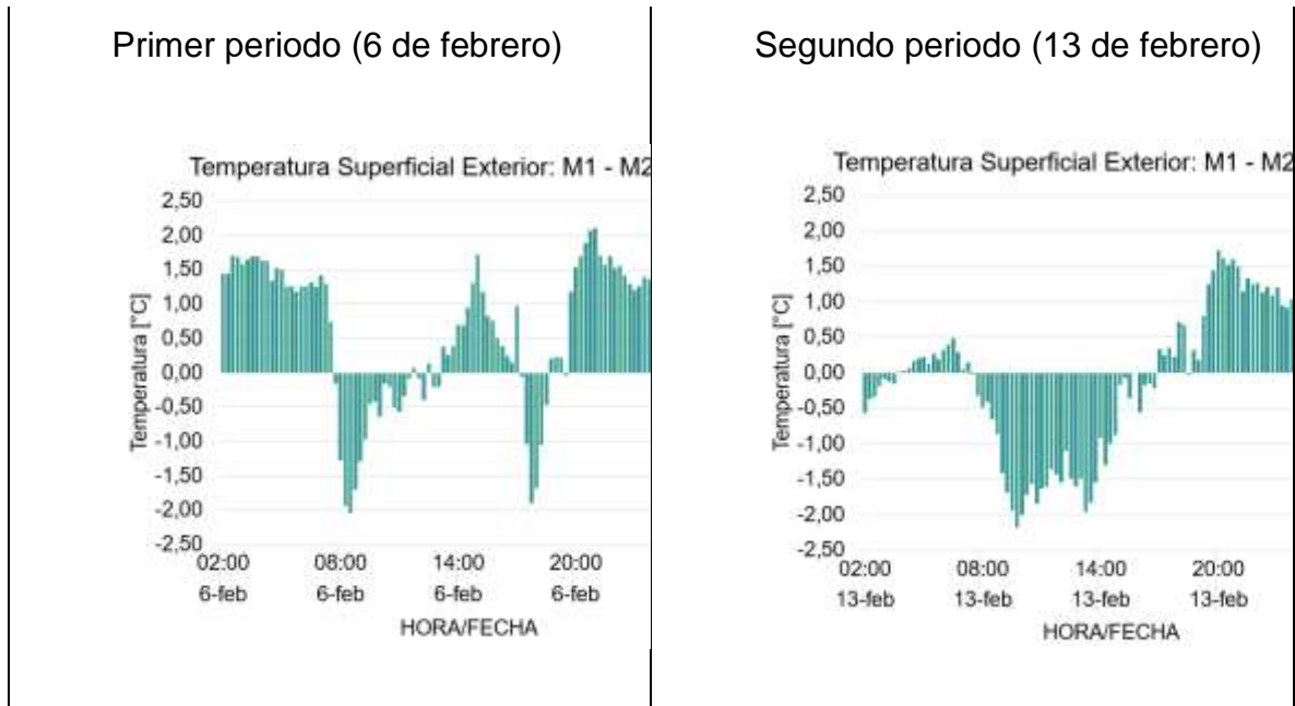
Figura 12. Diferencial hora a hora de la temperatura superficial exterior.
