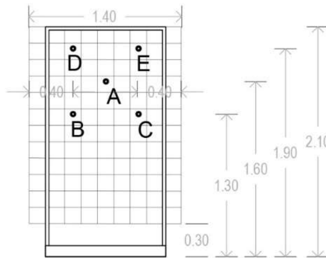
Figura 5. Puntos de medición de espesores.
