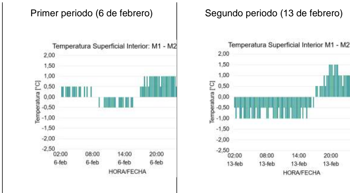
Figura 14. Diferencial hora a hora de la temperatura superficial interior.
