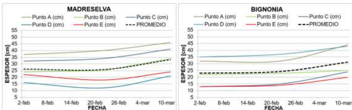
Figura 7. Espesores por punto y promedio.
