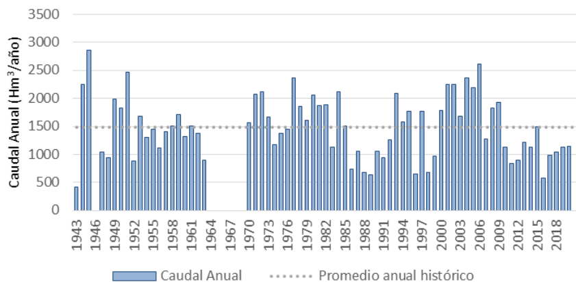
Figura 3: Análisis de caudales de la estación Los Altares, ubicada en la cuenca media del Río Chubut. Caudal anual (barras azules) y promedio anual histórico de caudales (línea punteada).
