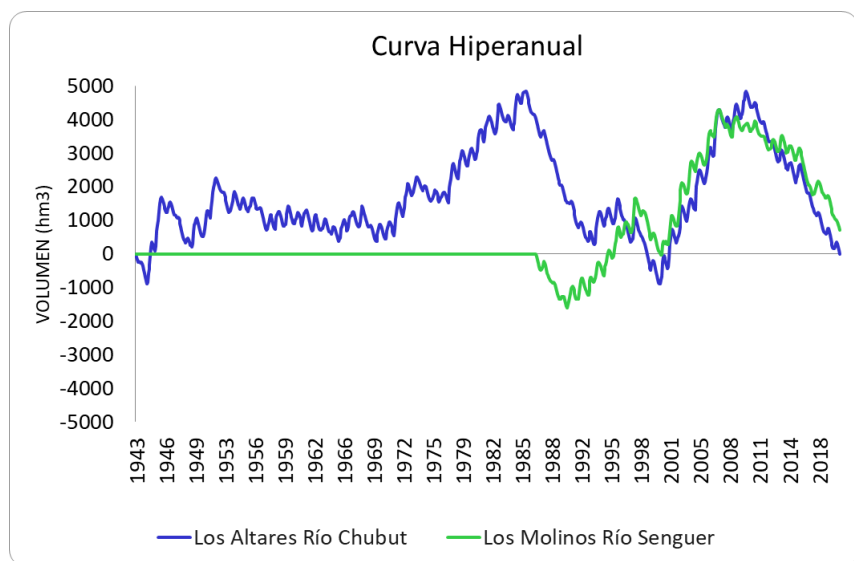
Figura 5. Curva de volúmenes acumulados abatidos o curva hiperanual (verde para Los Molinos sobre Río Senguer y azul para Los Altares sobre el Río Chubut). Los años con tendencia creciente corresponden a años con volúmenes de agua escurridos superiores al valor medio, marcando un periodo húmedo. Por el contrario, los años con tendencia decreciente corresponden a años con volúmenes de agua escurridos inferiores al valor medio, marcando un periodo seco.
