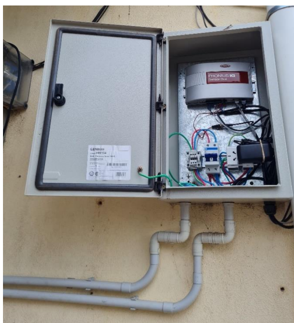
Figura 3a: Tablero para Sensor Box
