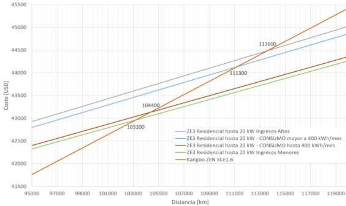
Figura 3. Evolución del costo acumulado para cada segmento tarifario en un escenario Kangoo ZE 3.
