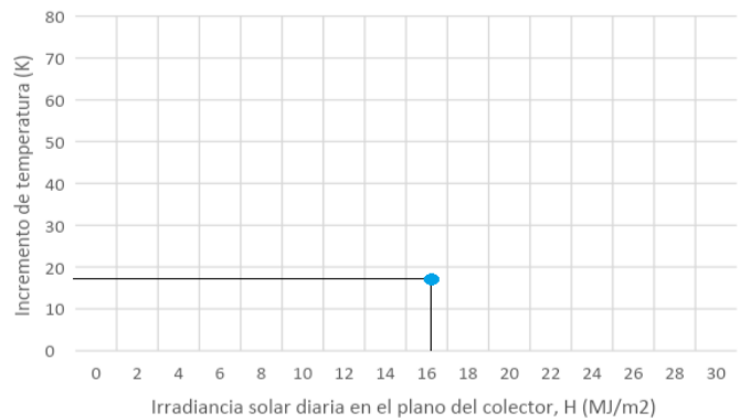
Figura 5. Diagrama de entrada en función de salida e incremento de la temperatura ensayo 22-08-23.
