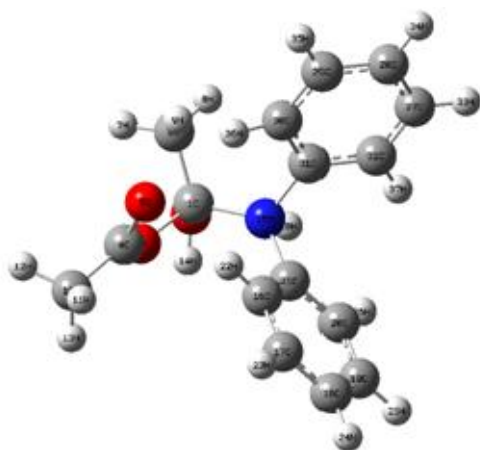
Figura 2.- Intermediario Tetraédrico
