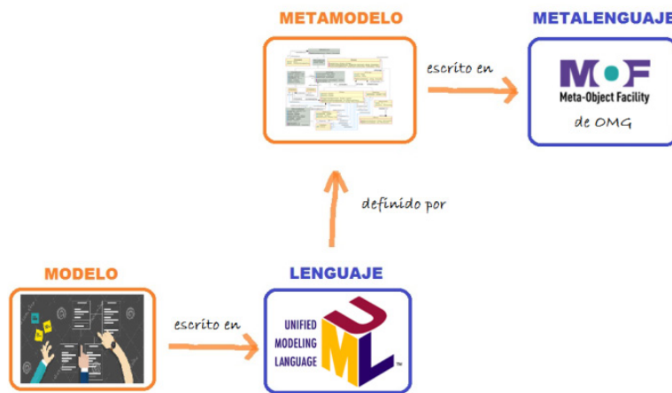
Figura 2: Modelo, Lenguaje, Metamodelos y Metalenguajes
