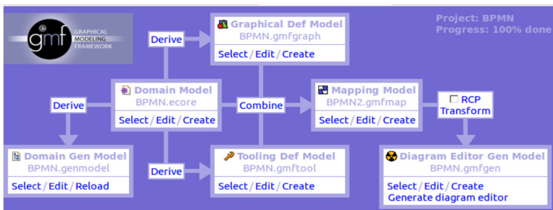
Figura 4: Dashboard del desarrollo de un proyecto GMF
