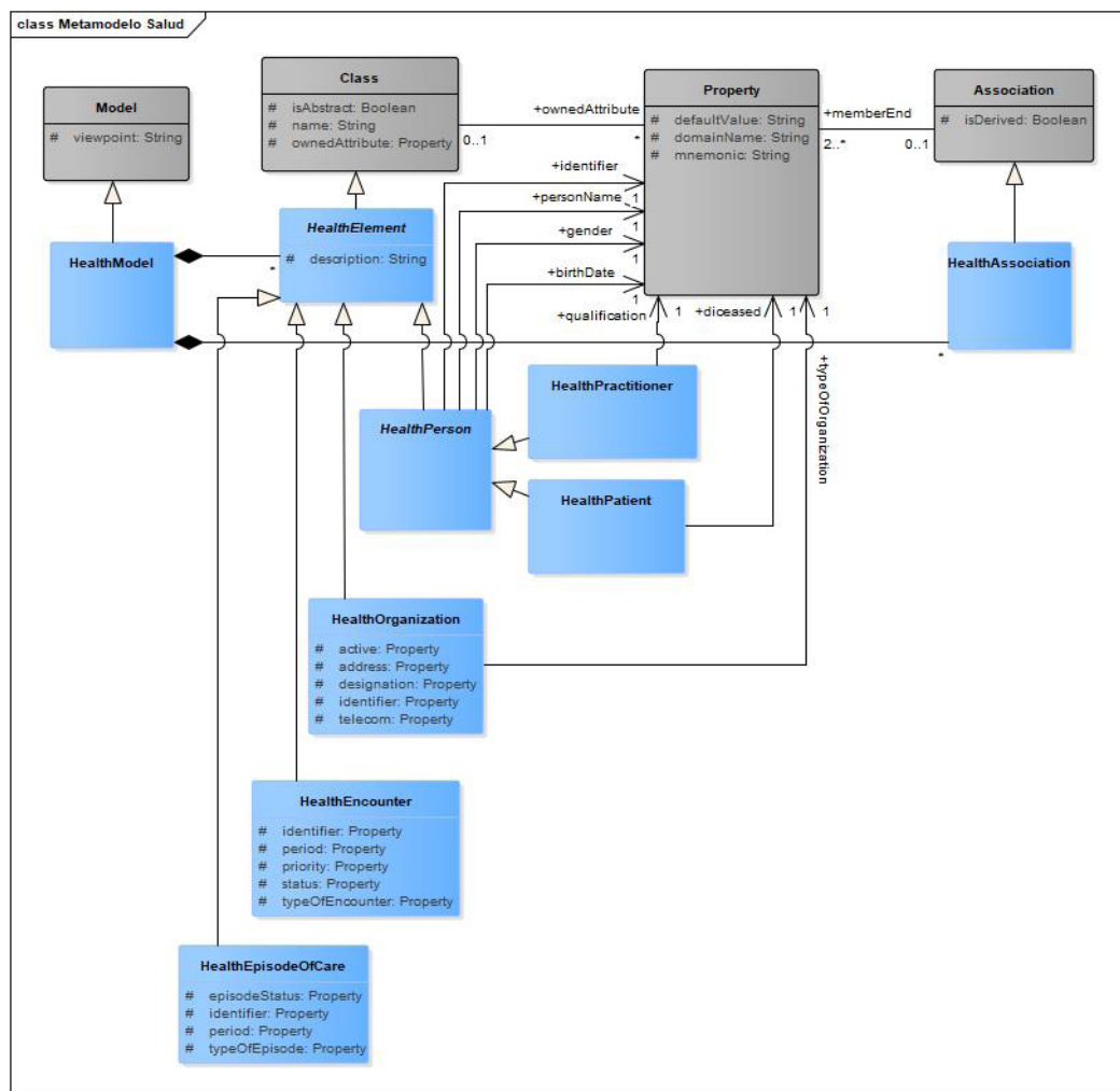
Figura 5: Metamodelo de Dominio Salud – DSL_SALUD
