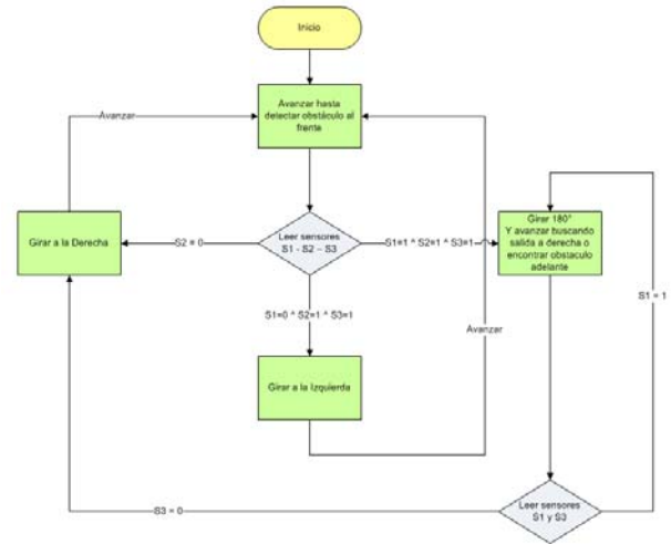
Fig. 8. Diagrama funcional del robot
