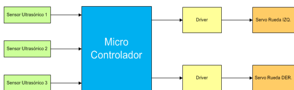
Fig. 1. Diagrama de bloques del robot
