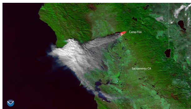
Figura 2: Imagen de incendio desde el NOAA-20.
