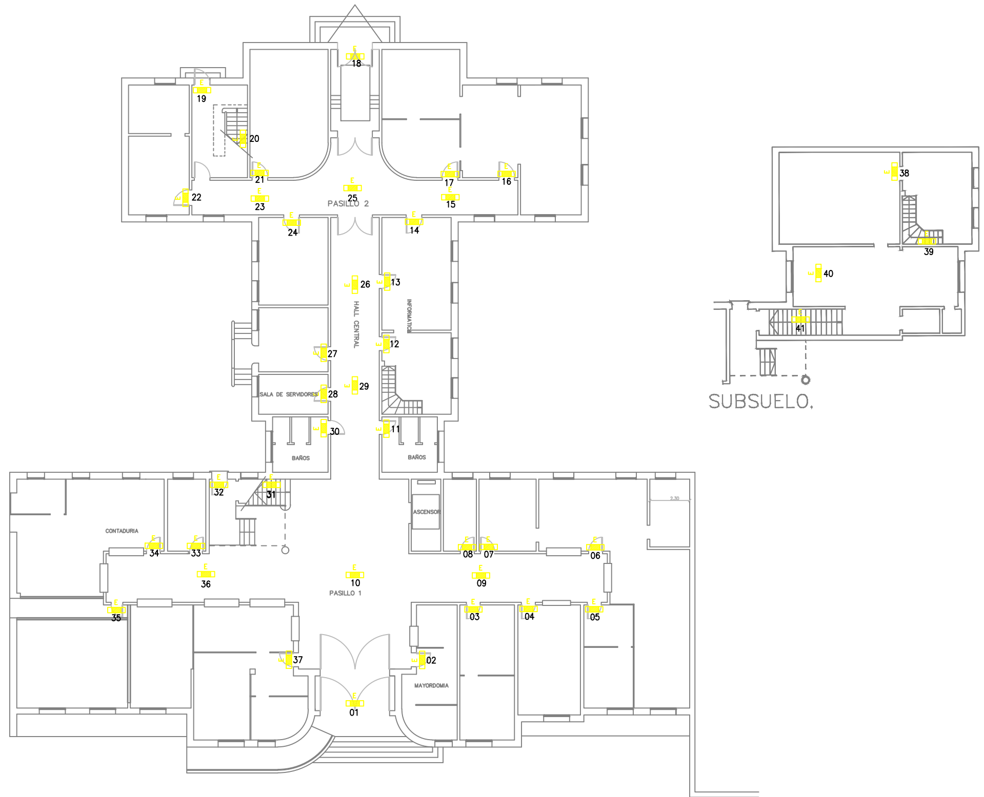
PLANO N°4 LUCES DE EMERGENCIA
