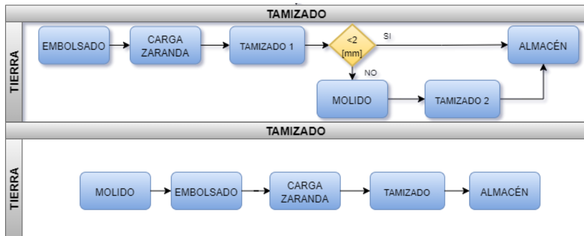
Figura 13: Metodología de trabajo actual (arriba) y nueva propuesta (abajo)
