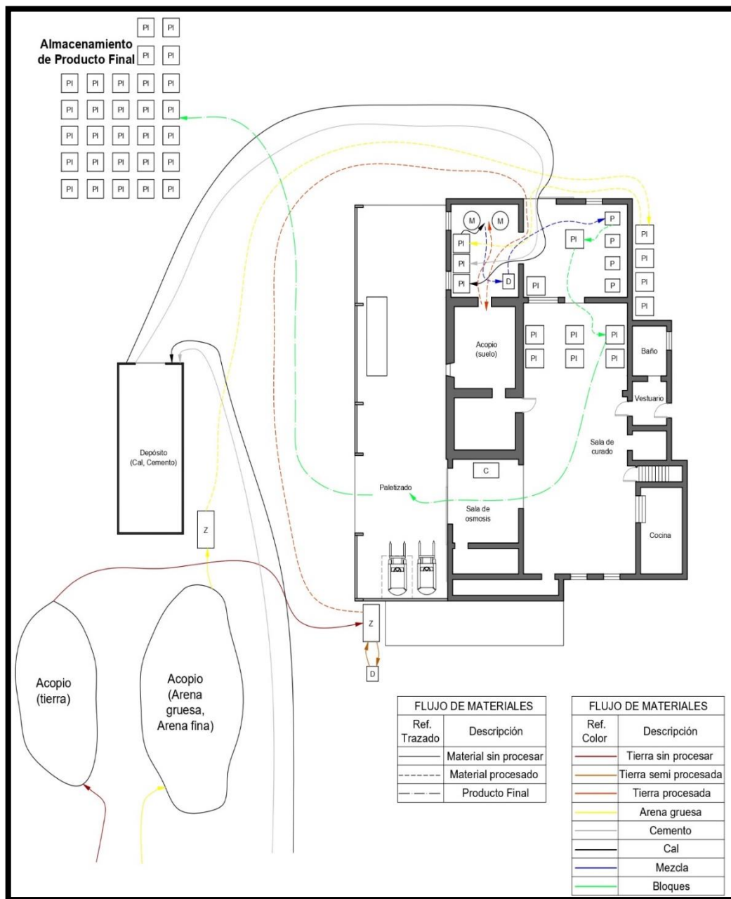
Figura 12: Distribución de equipos y sectores de GS Block
