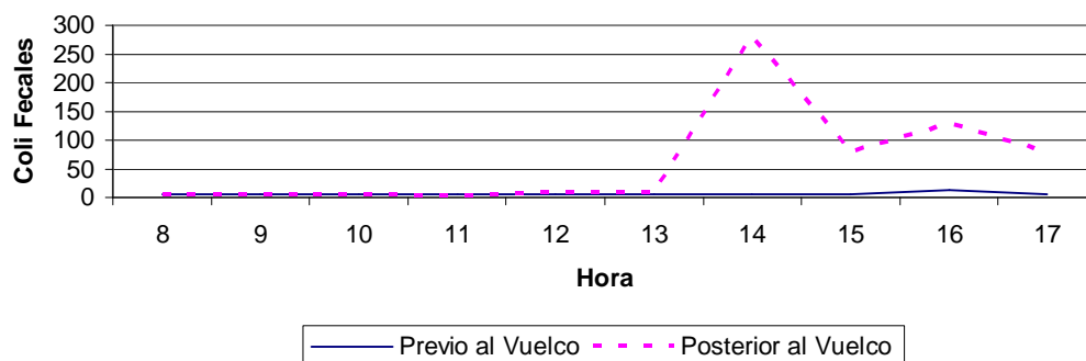
Figura N° 1 Variación temporal de los Coliformes Fecales antes y después del vuelco industrial del Frigorífico Las Camelias
