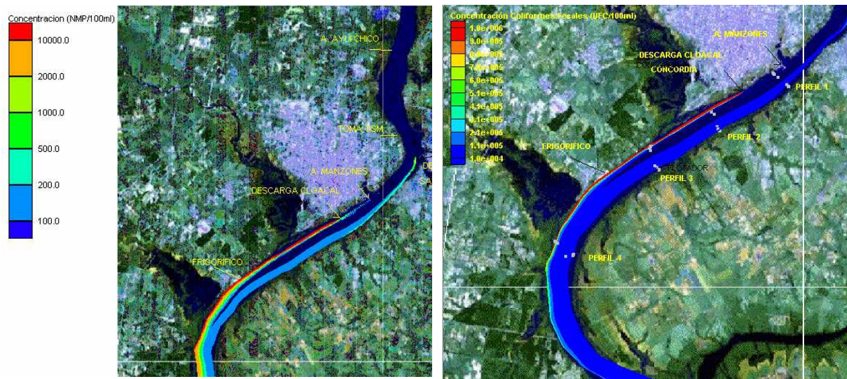
Figura N° 2 Vista general de la contaminación modelada considerando las descargas de Concordia y Salto (Rangos 100 a 10.000 y 10.000 a 1.000.000 UFC/100ml)
